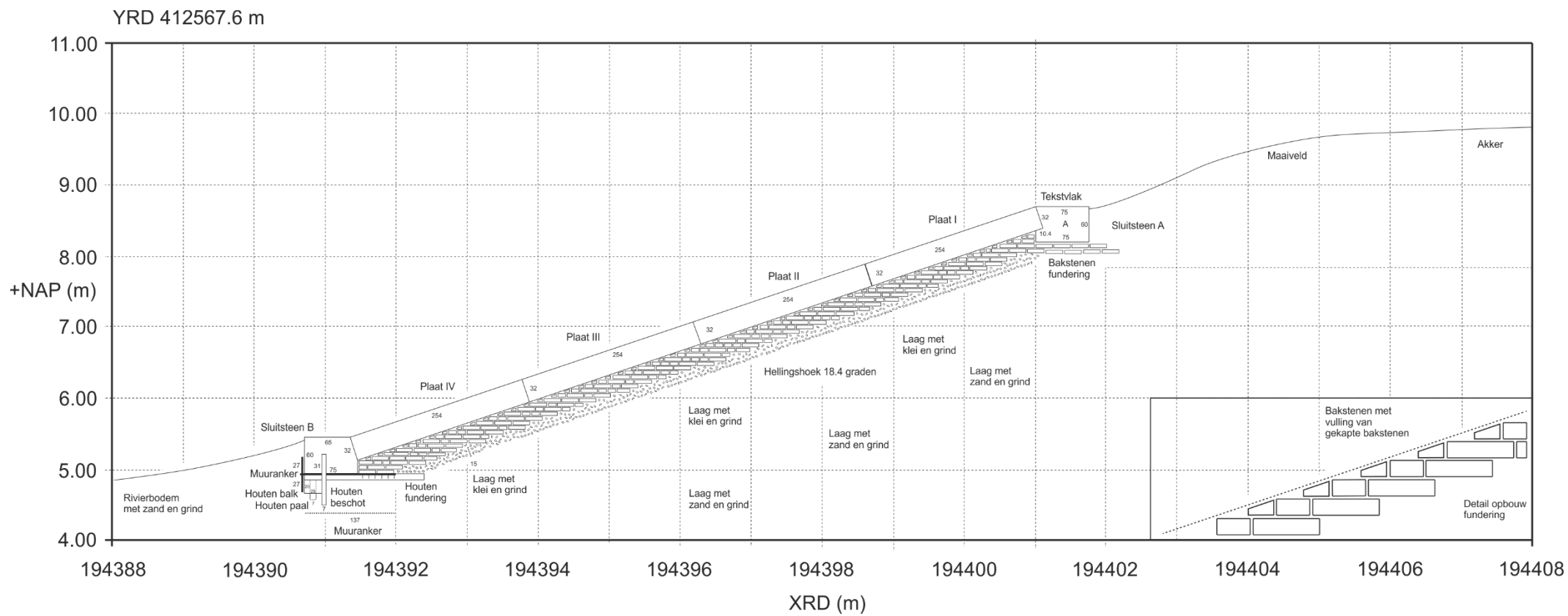
Afbeelding 15 De geogerefereerde projectie van het gereconstrueerde dwarsaanzicht, met afmetingen in centimeters.
