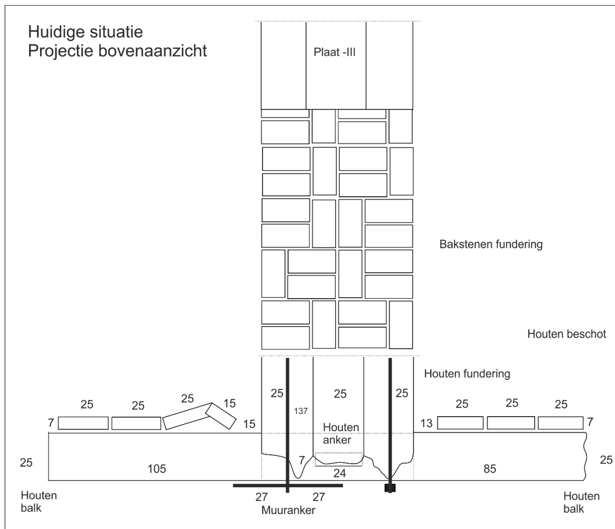
Afbeelding 10 Projectie van het huidige bovenaanzicht met afmetingen in centimeters.
